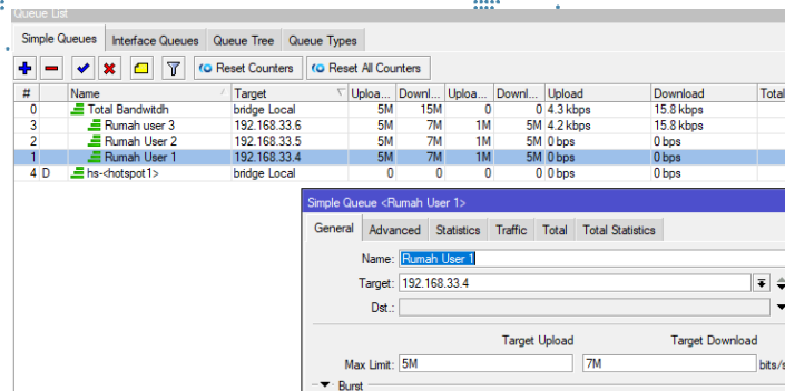
Gambar 6. Manajemen Bandwidth metode HTB
